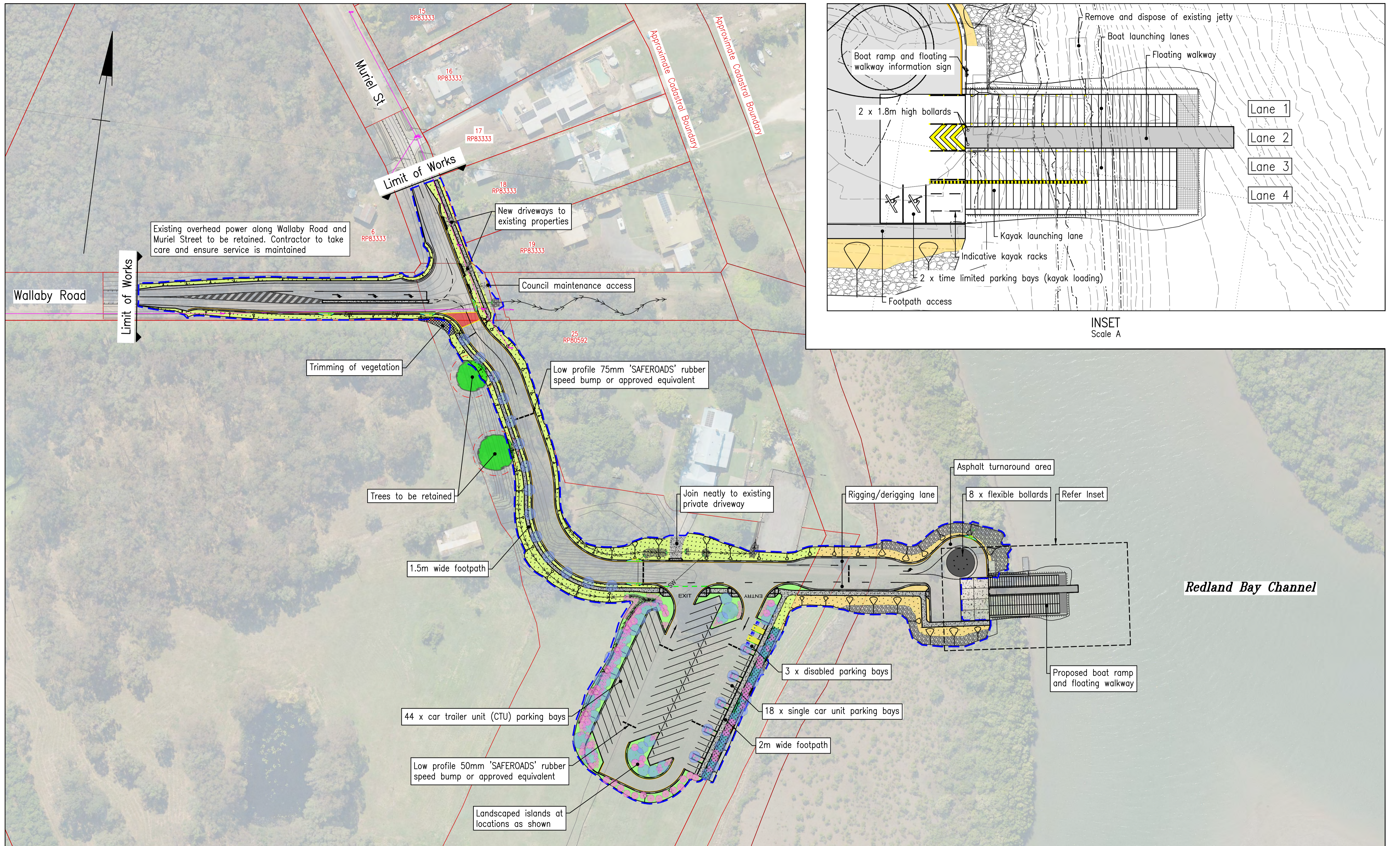
SITE PLAN NTS
