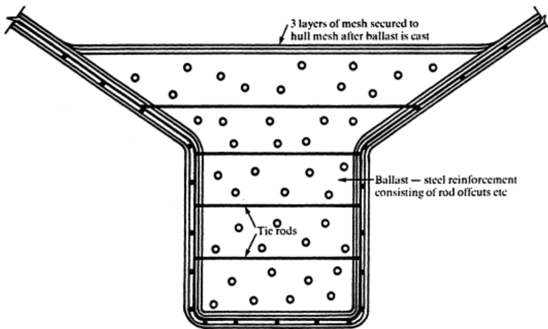
KEEL SECTION
